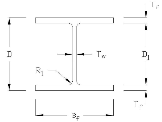
UNIVERSAL COLUMNS
